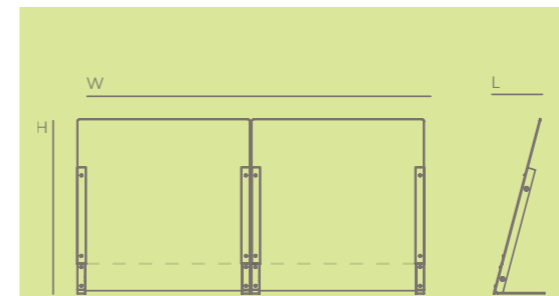
L10" W70" H29½" / 35 ½" L26cm W178cm H75cm / 90cm
