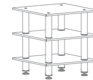
CLASSIC SMALL UNIT L29.5" W29.5" H35" L75cm W75cm H88.5cm
